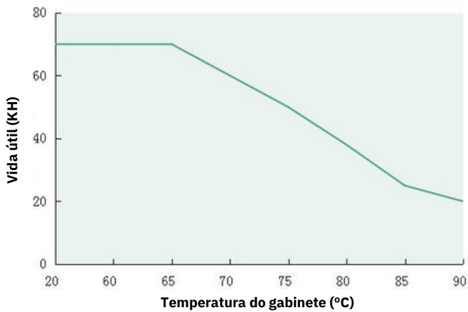
Tgabinete x Vida útil (DL-50H-MAL)
