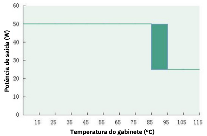
Potência de saída x Tgabinete (DL-50H-MAL)
