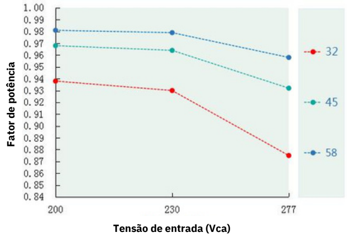
Fator de potência x Tensão de entrada (DL-50H-MAL)
