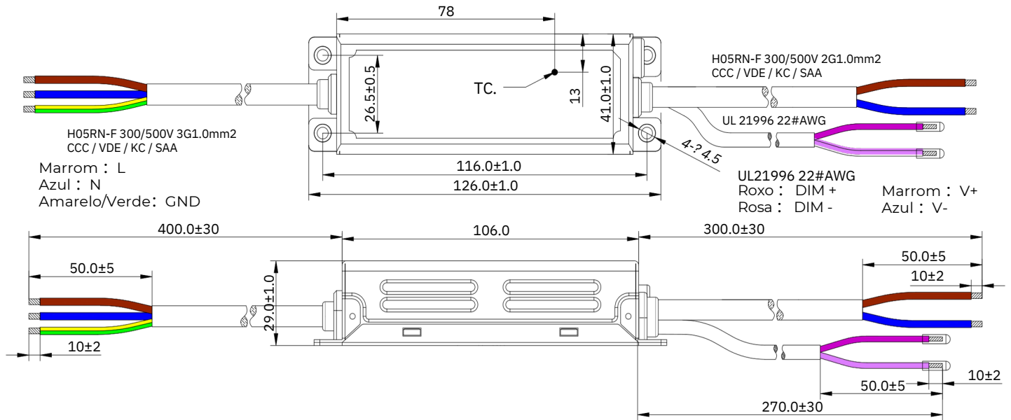
Desenho dimensional DL-50H-58S-MAL
