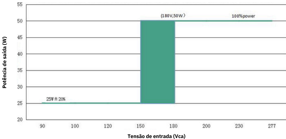
Potência de saída x Tensão de entrada DL-50H-58S-MAL. (Tensão de saída é 58 Vcc)
