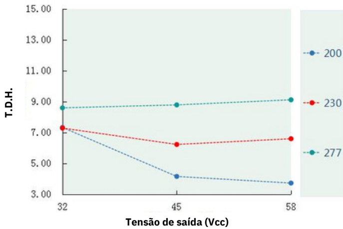
T.D.H. x Tensão de saída (DL-50H-MAL)
