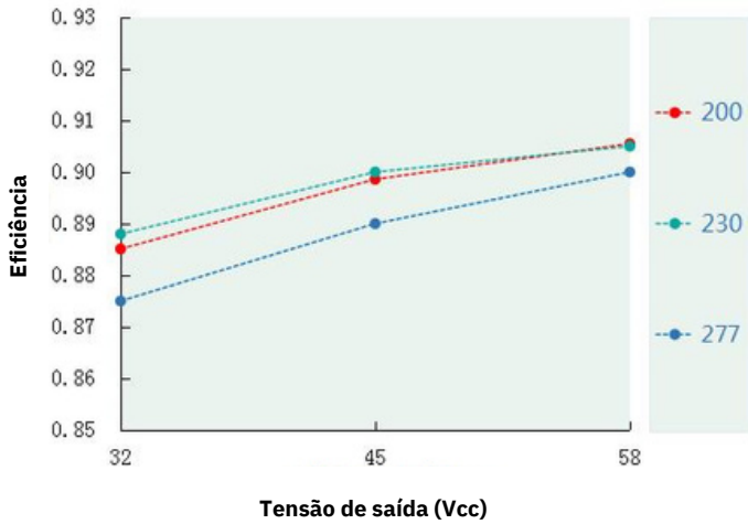
Rendimento x Tensão de saída (DL-50H-MAL)
